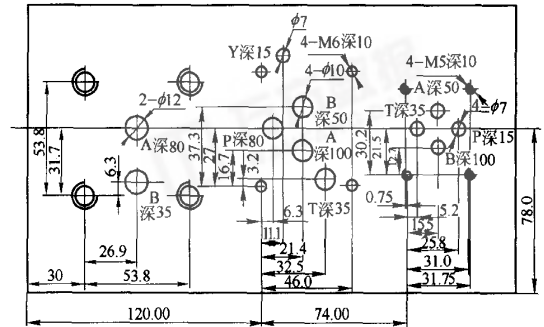
图3 液压阀块的主视图
