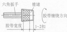
图1 缠锥堵
